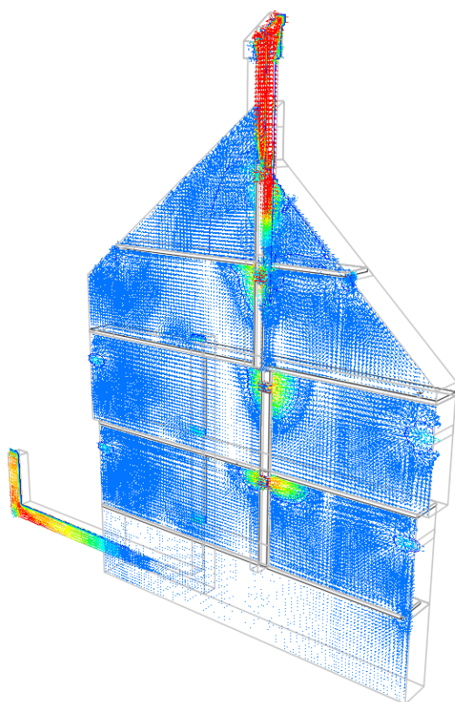
Byutvikling i Jugla-området, Riga, Latvia, utkast til arkitekturkonkurranse (2007), 11. posisjon. Modell av naturlig ventilasjon i en fleretasjes leilighetsbygning. Prosjektforslag i samarbeid med teknisk tegner N. Pettman og sivilingeniør J. Verhaegh.
